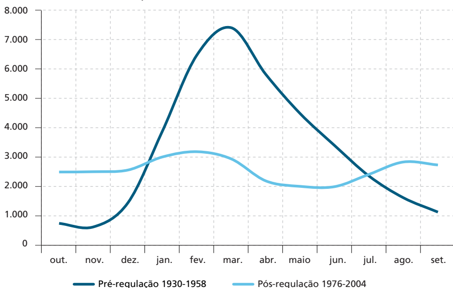
GRÁFICO 1 Vazão do rio Zambeze, média mensal em m 3 /s
