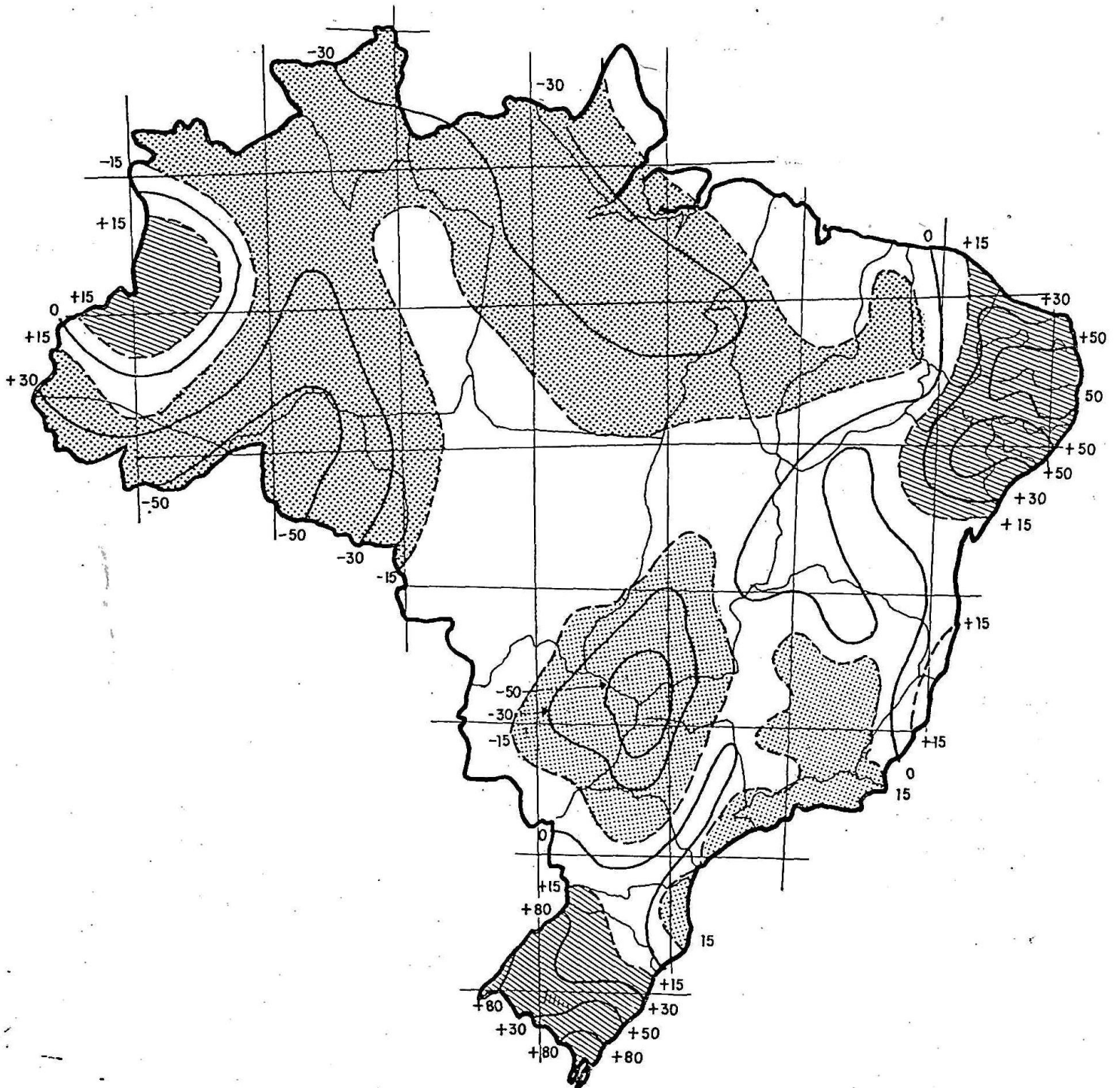
Figura 4 CURVA DE ISO-PRECIPITAÇÃO PARA 1914
