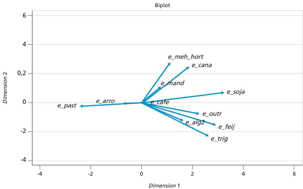
FIGURA 9 Diagrama bi-plot para efeitos-substituição – Minas Gerais (1995-2006)
