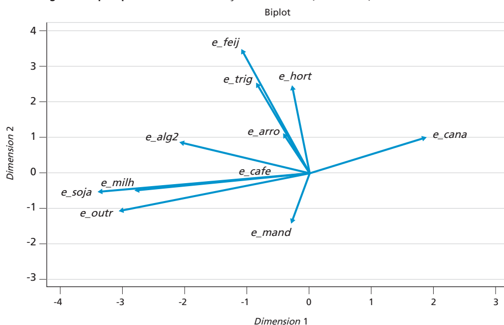
FIGURA 25 Diagrama bi-plot para efeitos-substituição – São Paulo (2006-2009)
