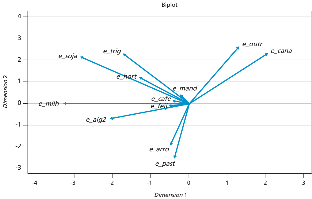
FIGURA 24 Diagrama bi-plot para efeitos-substituição – São Paulo (1995-2006)
