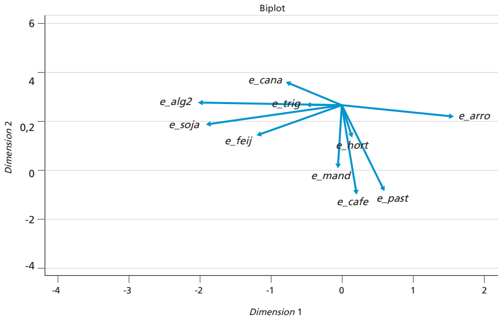
FIGURA 12 Diagrama bi-plot para efeitos-substituição – Mato Grosso (1995-2006)
