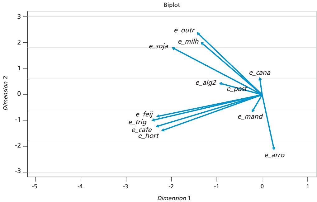
FIGURA 21 Diagrama bi-plot para efeitos-substituição – Goiás (1995-2006)
