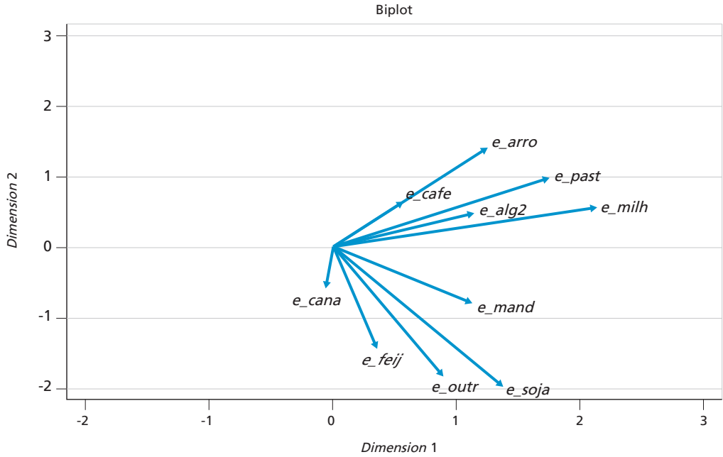
FIGURA 18 Diagrama bi-plot para efeitos-substituição – Tocantins (1995-2006)
