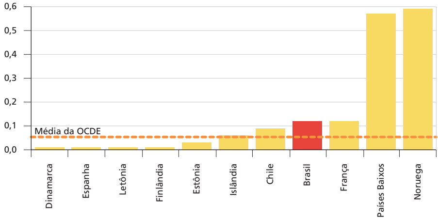
GRÁFICO 21 Receita tributária relacionada ao oceano como parcela da receita tributária total (Em %)
