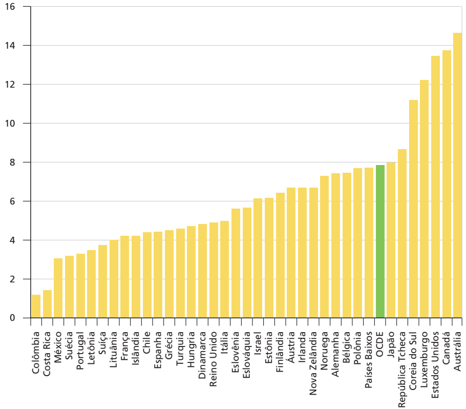
GRÁFICO 10 Intensidade de emissões do uso da energia per capita (2021) (Em toneladas de CO 2 per capita )
