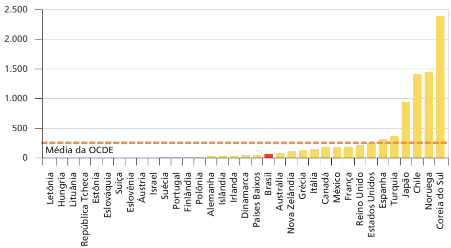
GRÁFICO 26 Brasil versus membros da OCDE: produção total da aquicultura, espécies marinhas e parcialmente marinhas (2019) (Em 1 mil toneladas)
