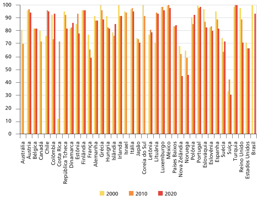
GRÁFICO 15 Receita fiscal da poluição do ar (2000-2020) (Em % da receita fiscal relacionada a meio ambiente)
