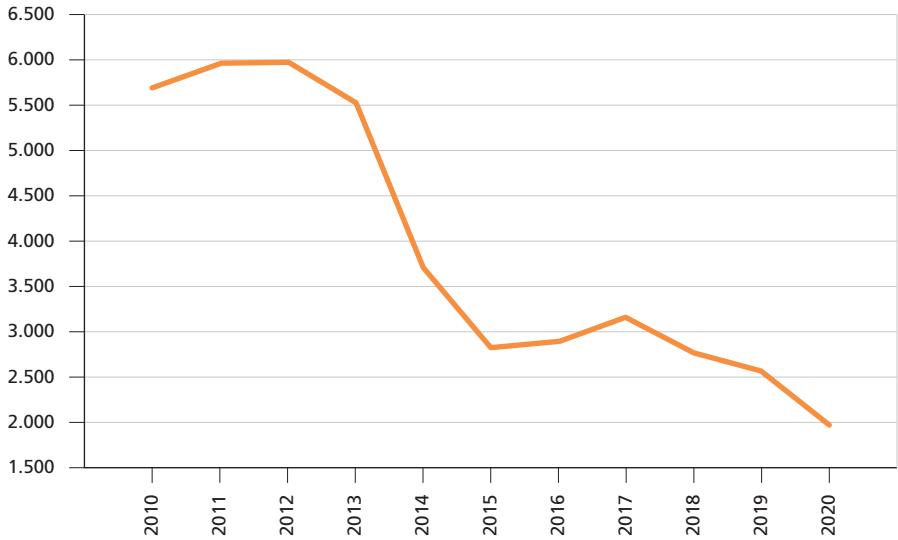
GRÁFICO 23 Brasil: medidas de apoio a combustíveis fósseis relacionados ao oceano beneficiando produtores (PSE) (2010-2020) (Em US$ milhões nominais)
