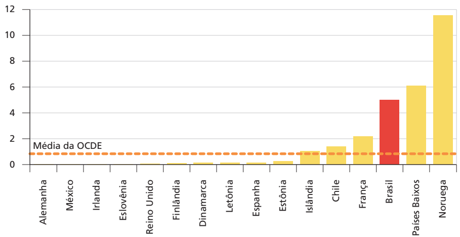
GRÁFICO 19 Receita tributária relacionada ao oceano como parcela da receita tributária ambiental (Em %)
