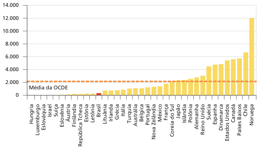
GRÁFICO 30 Exportações totais de produtos pesqueiros (2019) (Em US$ milhões)
