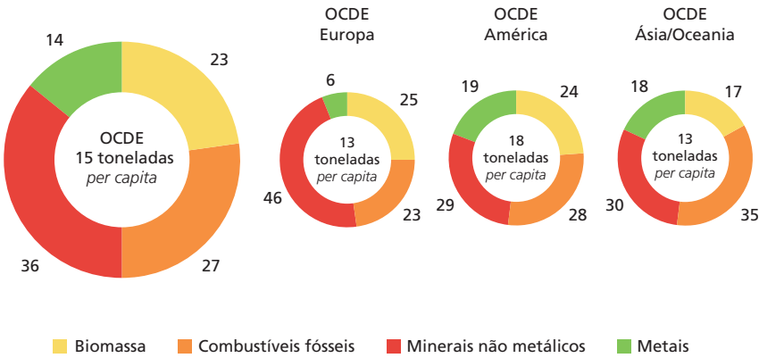
GRÁFICO 6 Mix de materiais consumidos no âmbito da OCDE (2017) (Em toneladas per capita )
