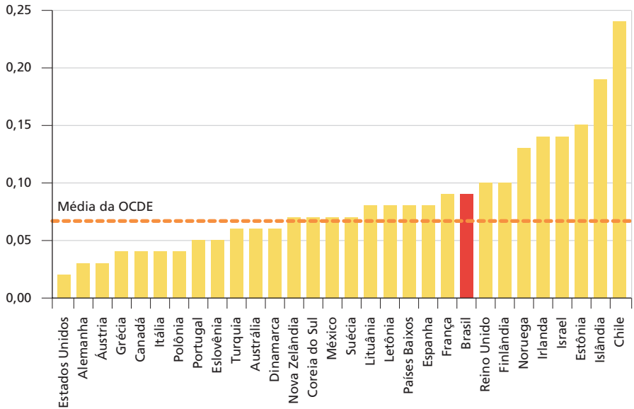
GRÁFICO 16 Número de instrumentos de política relacionados ao oceano como parte de todos os instrumentos de política
