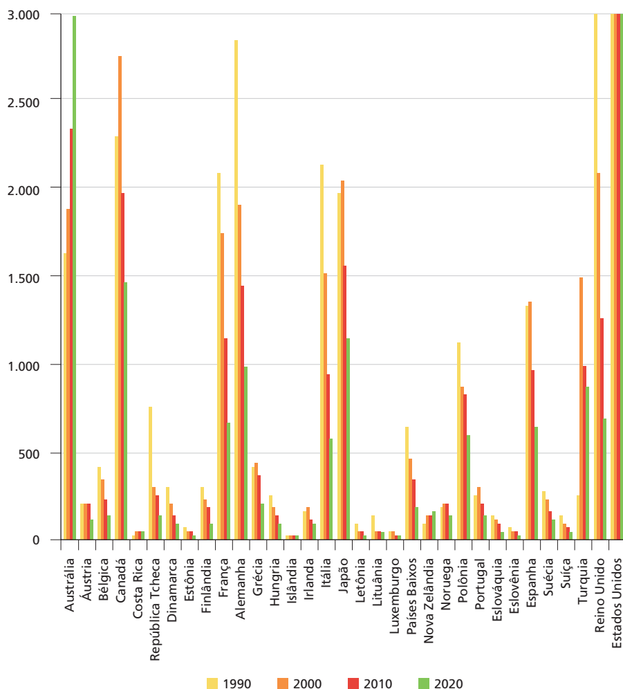
GRÁFICO 7 Emissões de NO x (1990-2020) (Em milhares de toneladas)
