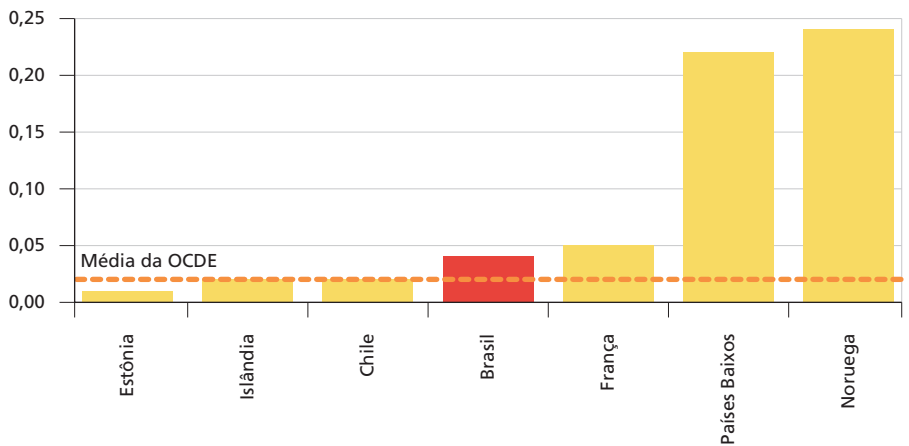
GRÁFICO 20 Receita tributária relacionada ao oceano como parcela do PIB (Em %)
