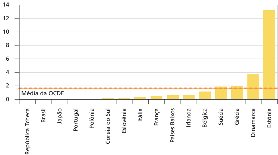
GRÁFICO 34 Receitas do transporte marítimo internacional de passageiros como parcela das receitas totais do turismo internacional (Em %)
