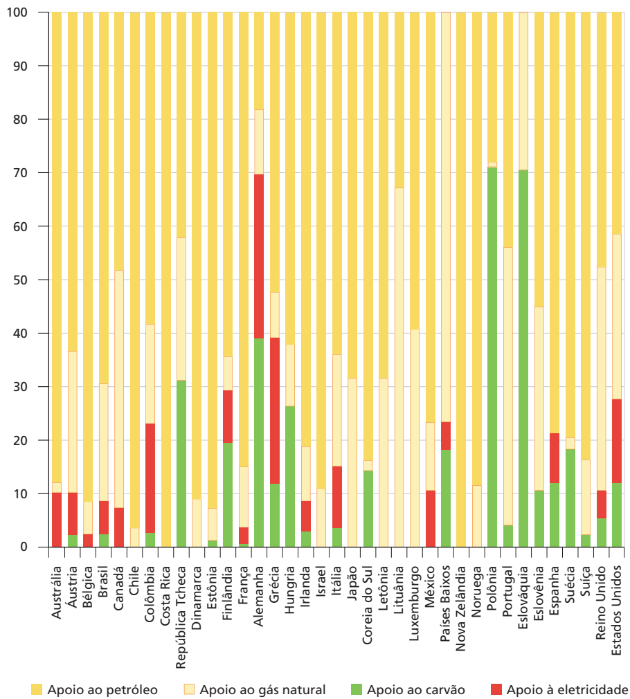
GRÁFICO 27 Tipo de combustível beneficiado pelas medidas de apoio aos combustíveis fósseis (2021) (Em %)
