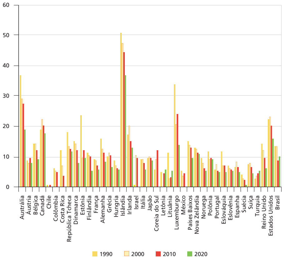
GRÁFICO 7 Emissões totais de GEEs incluindo o setor LULUCF per capita (1990-2020) (Em toneladas de CO 2 e per capita )
