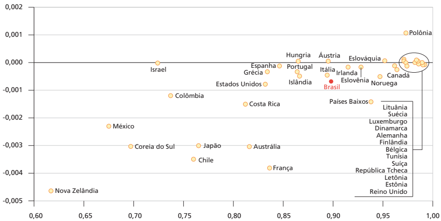
GRÁFICO 5 Índice da Lista Vermelha (2021) versus tendência linear (2001-2021)
