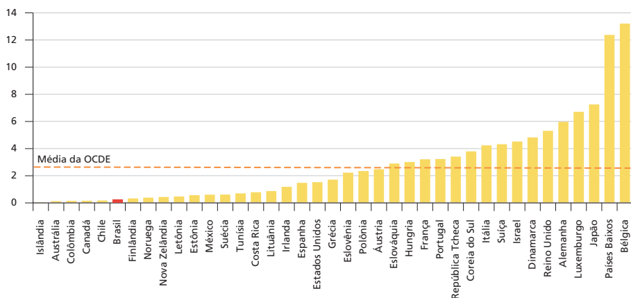
GRÁFICO 2 Áreas construídas no total do território (2000) (Em %)
