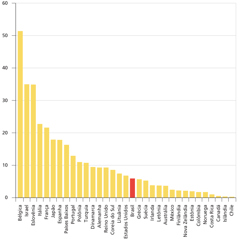
GRÁFICO 1 Brasil versus membros da OCDE: área construída dentro de 1 km da costa como porcentagem da terra dentro de 1 km da costa (2014) (Em %)
