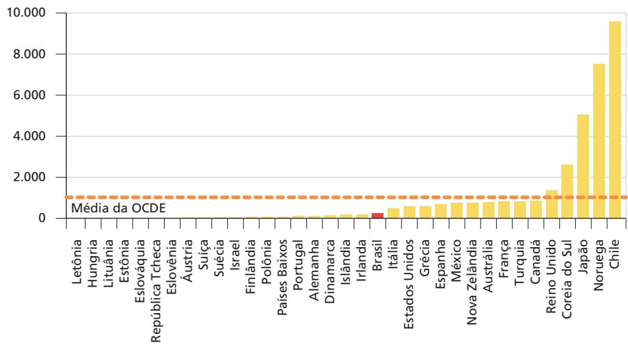
GRÁFICO 25 Produção aquícola total, espécies marinhas e parcialmente marinhas (Em US$ milhões)
