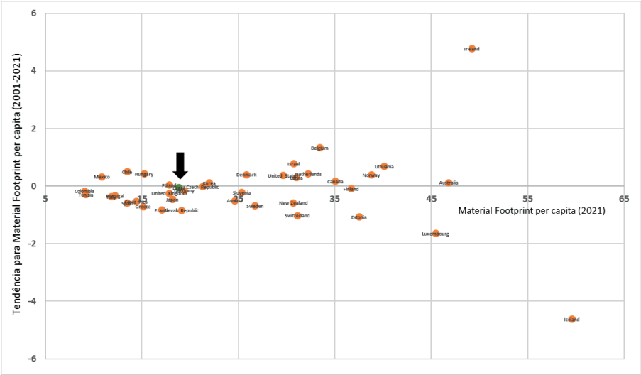
FIGURA 3 Mapa perceptual para confrontar a pegada material per capita em 2021 com a sua tendência de crescimento nos países da OCDE e do Brasil em 2001-2021
