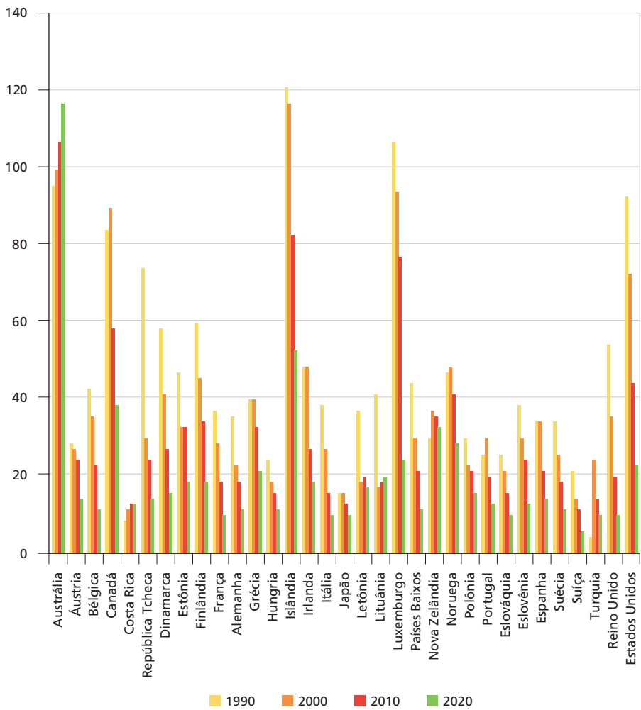
GRÁFICO 8 Emissões de NO x per capita (1990-2020) (Em NO x kg/capita)
