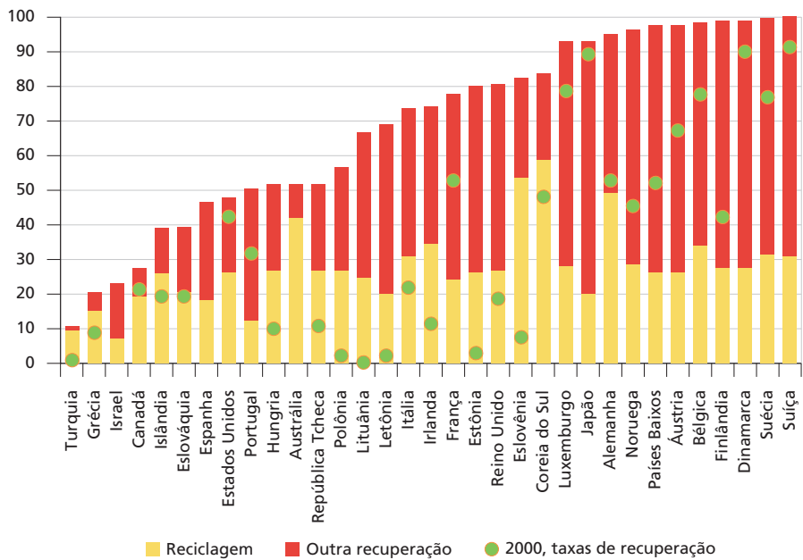
GRÁFICO 2 Reciclagem e taxa de recuperação de resíduos no âmbito dos países da OCDE (Em %)
