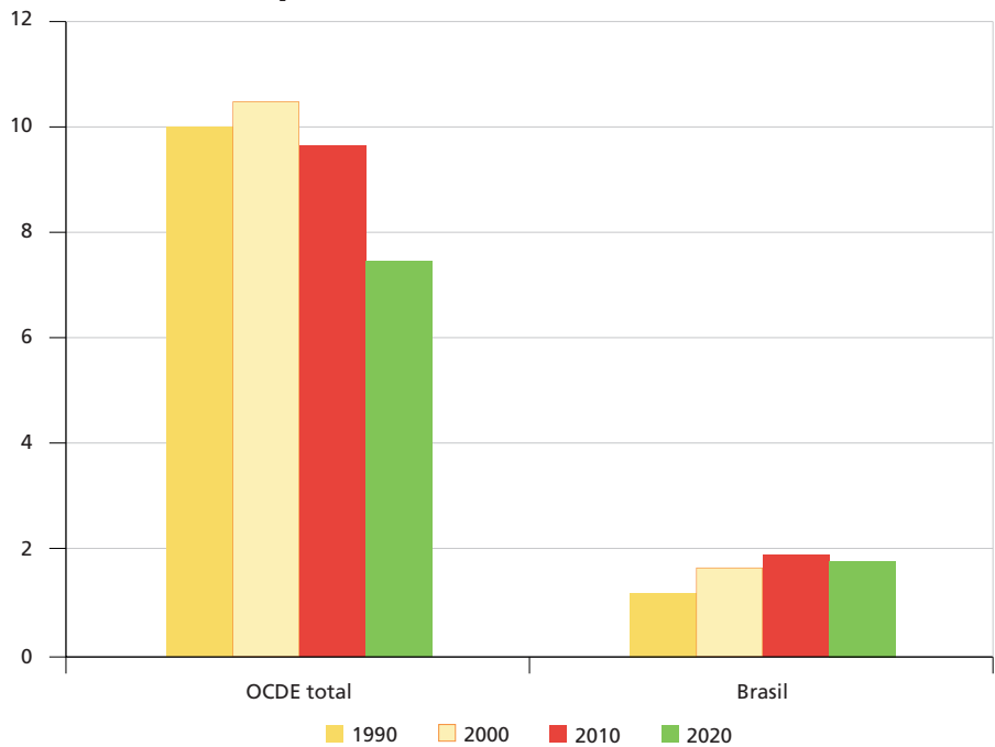
GRÁFICO 11 Intensidade de emissões do uso da energia per capita (1990-2020) (Em toneladas de CO 2 per capita )
