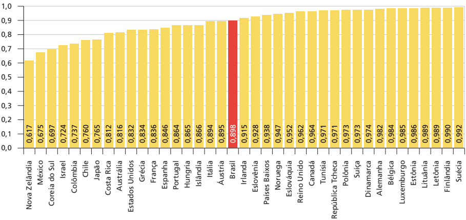
GRÁFICO 4 Índice da Lista Vermelha (2021)
