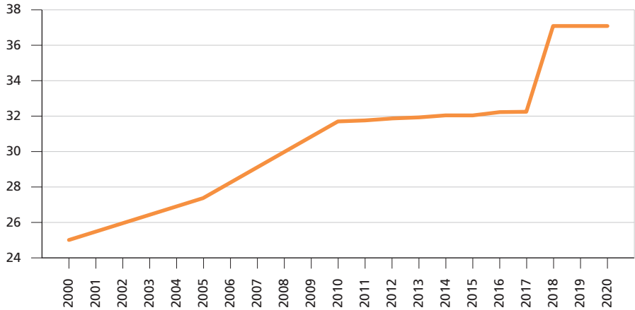
GRÁFICO 14 Brasil: MPA total dentro de 10 km da costa (tanto terrestre quanto marinha) como parte da área tampão de 10 km (2000-2020) (Em %)
