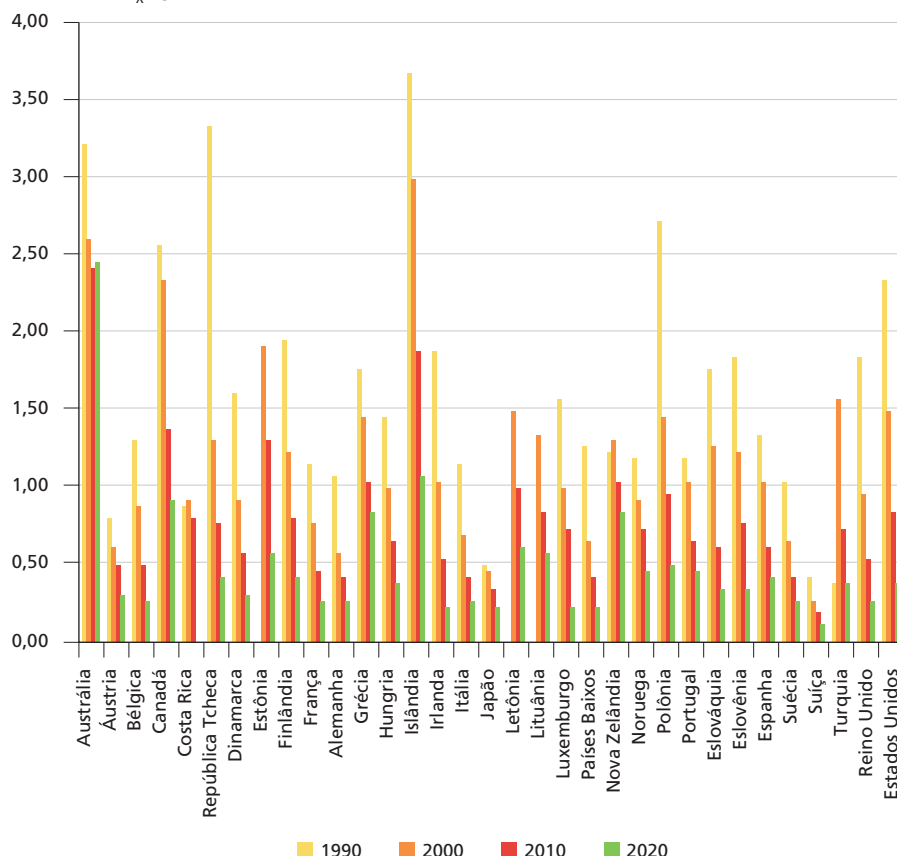
GRÁFICO 9 Intensidade de NO x do PIB (1990-2020) (Em NO x kg/US$ 1 mil)
