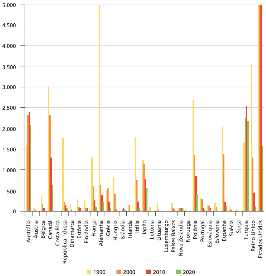
GRÁFICO 4 Emissões totais de SO x (1990-2020) (Em milhares de toneladas)
