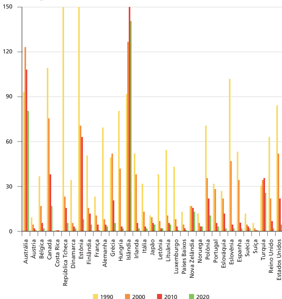
GRÁFICO 5 Emissões de \text{SO}_x per capita (1990-2020) (Em \text{SO}_x kg/capita)
