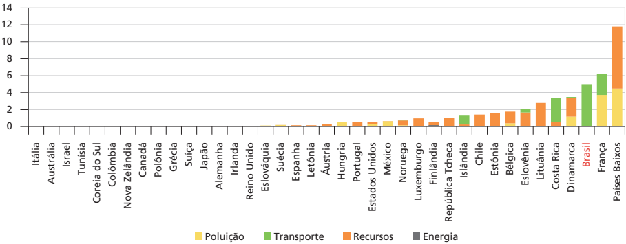
GRÁFICO 9 Receita tributária relacionada à biodiversidade por base tributária (2019) (Em % total da tributação ambiental)
