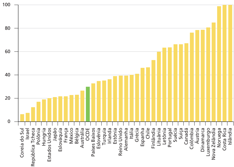
GRÁFICO 21 Parcela de fontes renováveis na produção de eletricidade (2021) (Em %)
