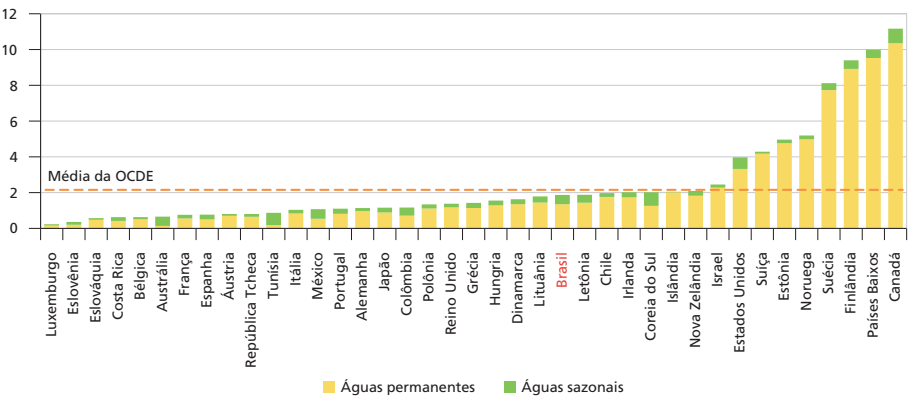
GRÁFICO 3 Superfícies permanentes e sazonais no total da superfície de água: porcentagem no total da área do país (2015)
