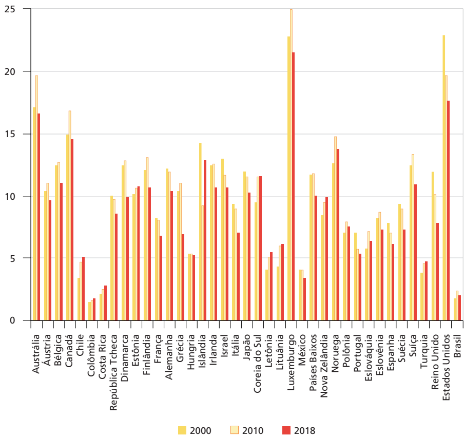
GRÁFICO 15 Emissões de CO 2 do uso da energia da demanda doméstica per capita (2000-2018) (Em toneladas de CO 2 per capita )
