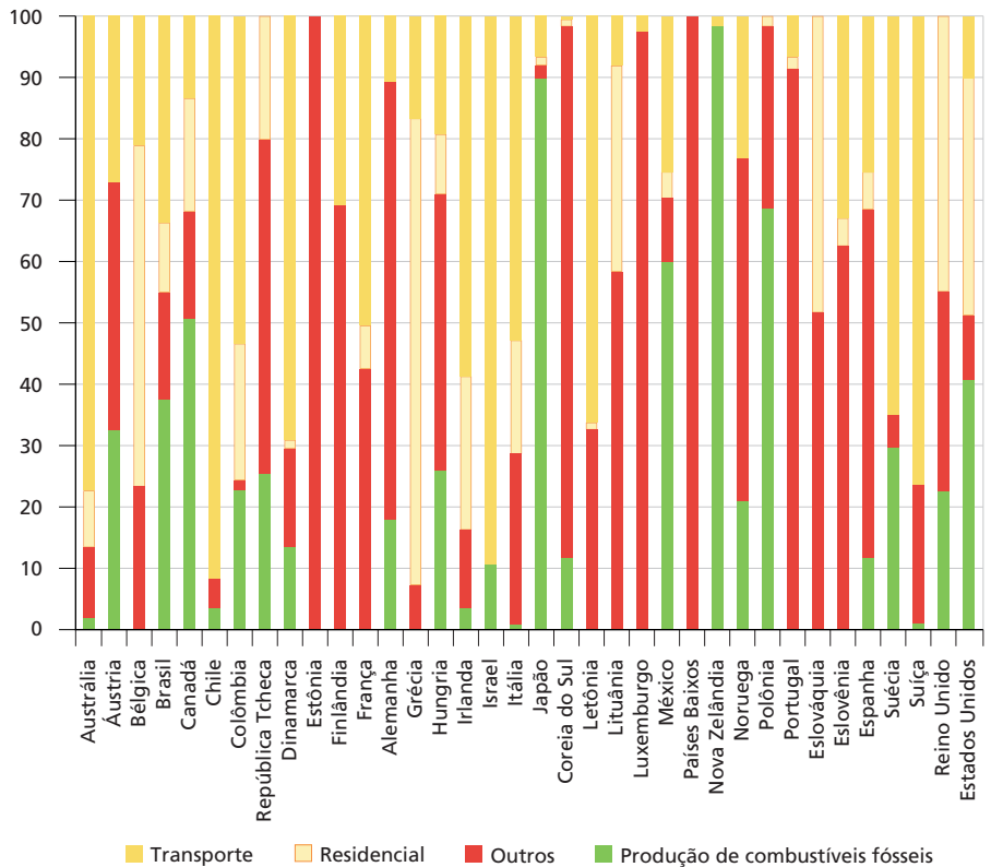
GRÁFICO 29 Medidas de apoio aos combustíveis fósseis por setores beneficiados (2021) (Em %)
