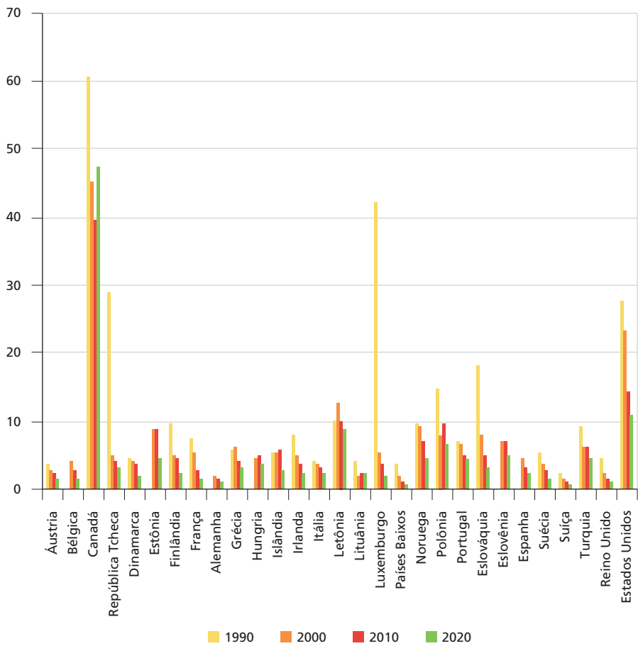
GRÁFICO 2 Emissões de PM 2.5 per capita (1990-2020) (Em PM 2.5 kg/capita)
