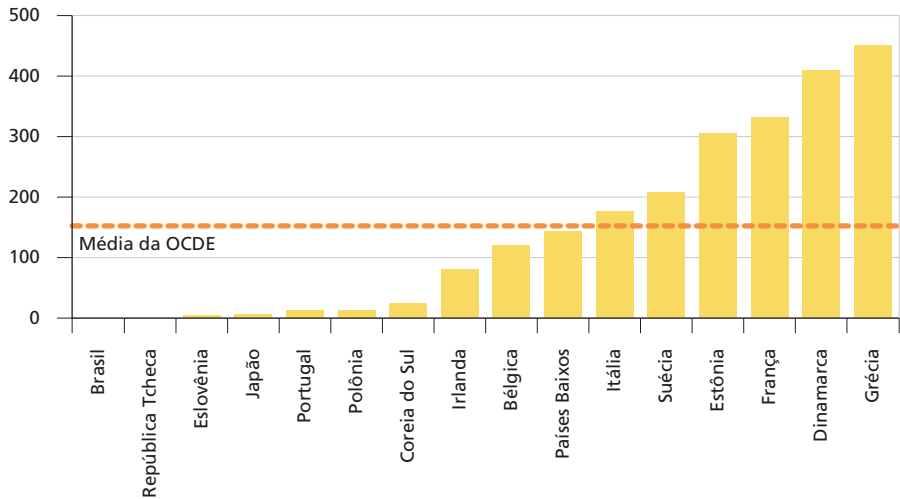
GRÁFICO 35 Receitas de transporte marítimo internacional de passageiros (2019) (Em US$ milhões)
