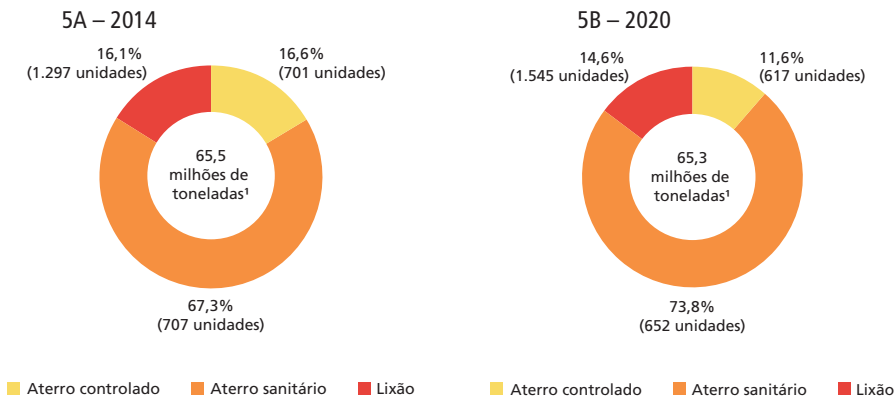
GRÁFICO 5 Brasil: estimativas da disposição final de resíduos urbanos (2014 e 2020)
