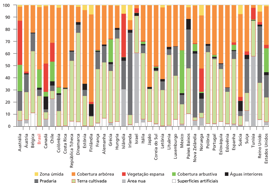
GRÁFICO 1 Cobertura da terra por tipo (2019) (Em %)
