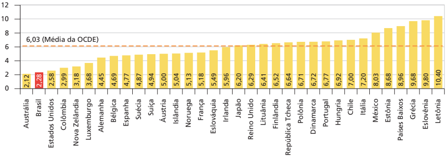
GRÁFICO 11 Receita tributária relacionada a meio ambiente (2020) (Em % total da receita tributária)
