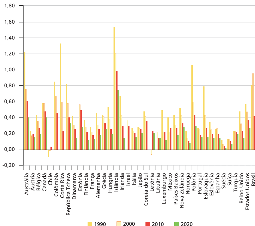
GRÁFICO 8 Intensidade de GEEs do PIB (1990-2020) (Em tCO 2 e/US$ 1 mil)
