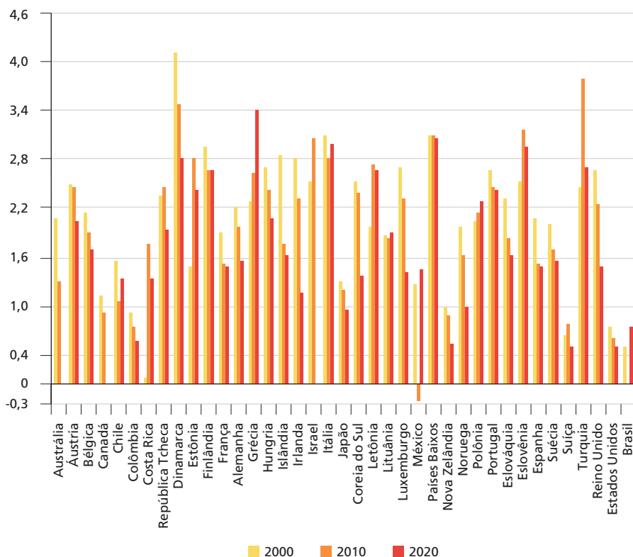
GRÁFICO 14 Receita fiscal da poluição do ar (2000-2020) (Em % do PIB)
