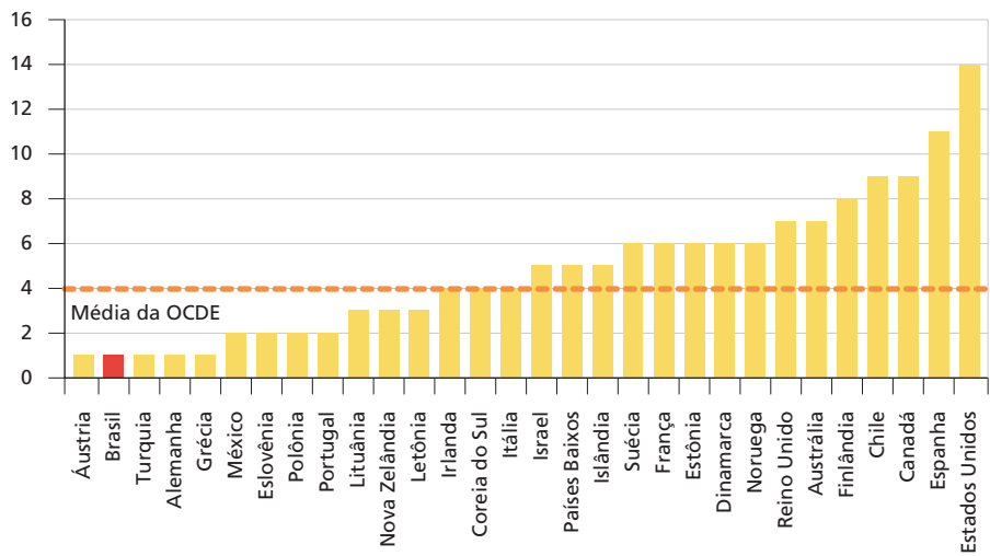
GRÁFICO 17 Número de instrumentos de política relacionados ao oceano
