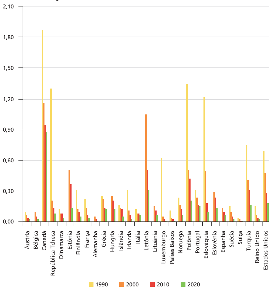
GRÁFICO 3 Intensidade de PM 2.5 do PIB (1990-2020) (Em PM 2.5 kg/US$ 1 mil)
