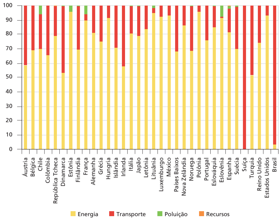
GRÁFICO 17 Receita fiscal da poluição do ar, por setor (2020) (Em % da receita fiscal relacionada a meio ambiente)
