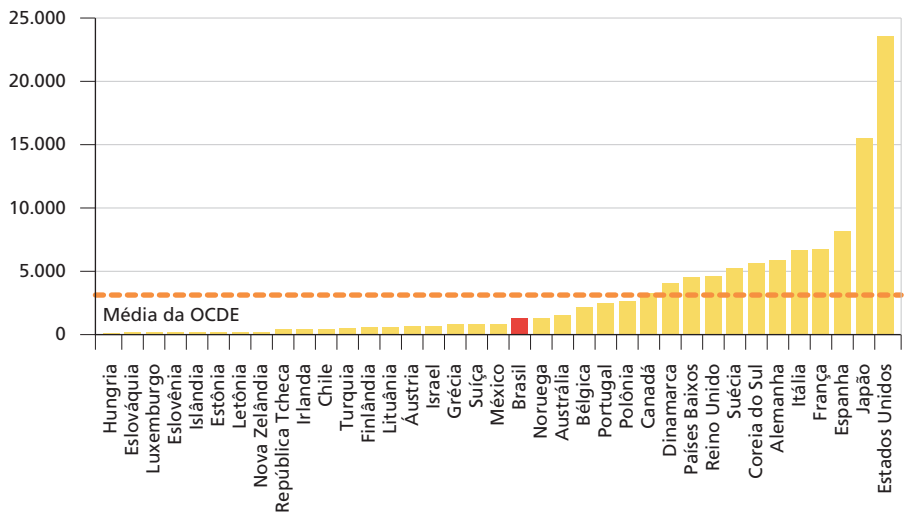
GRÁFICO 31 Importações totais de produtos da pesca (2019) (Em US$ milhões)
