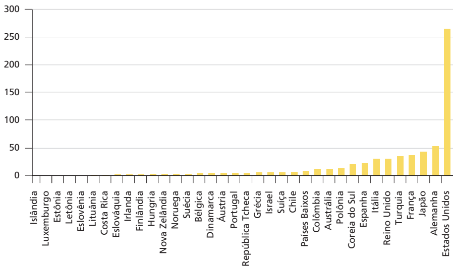
GRÁFICO 3 Dados dos países da OCDE para resíduos urbanos 3A – Em 1 mil toneladas
