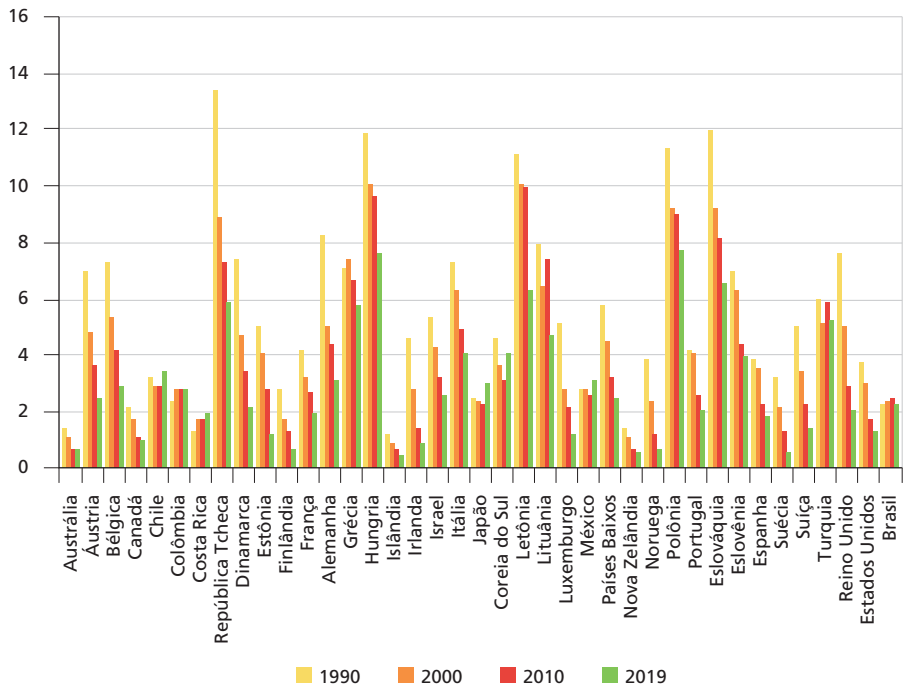
GRÁFICO 13 Custo da mortalidade por PM 2.5 (1990-2020) (Em % do PIB equivalente)
