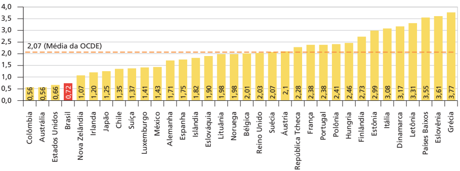
GRÁFICO 10 Receita tributária relacionada a meio ambiente (2020) (Em % do PIB)
