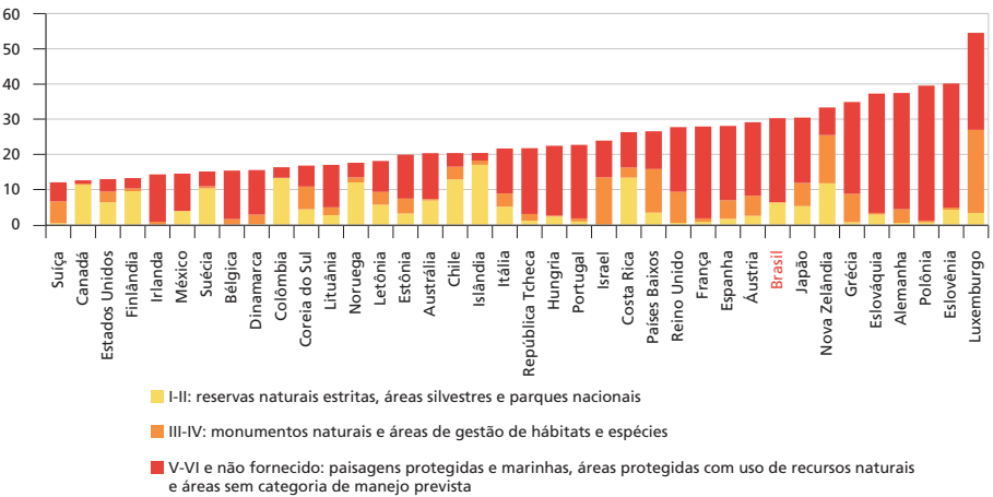
GRÁFICO 6 Área terrestre protegida por tipo (2022) (Em % da área total)
