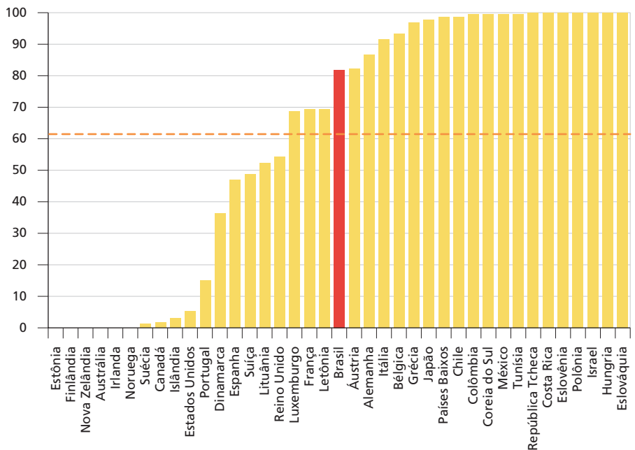
GRÁFICO 11 População exposta a concentrações de PM 2.5 superiores a 10 mcg/m 3 (2019) (Em %)
