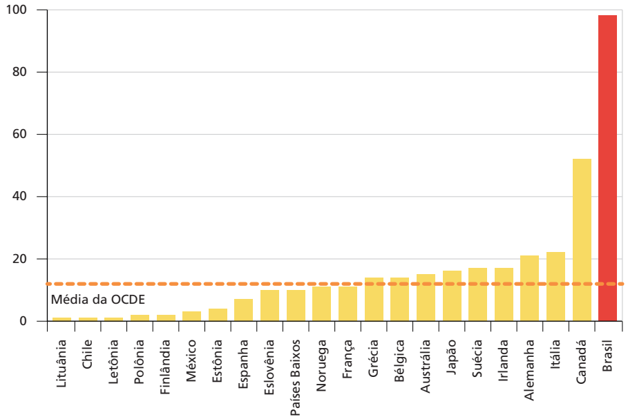
GRÁFICO 4 Espécies de peixes marinhos ameaçadas
