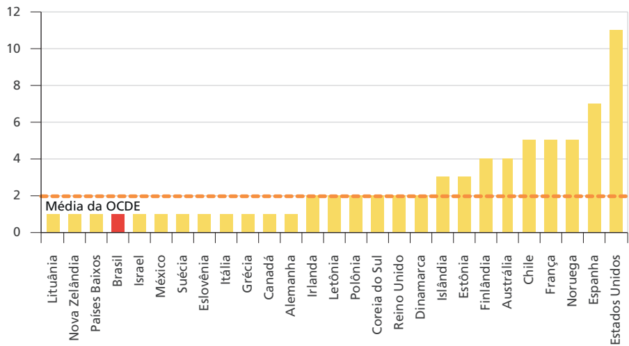
GRÁFICO 18 Número de impostos relacionados ao oceano
